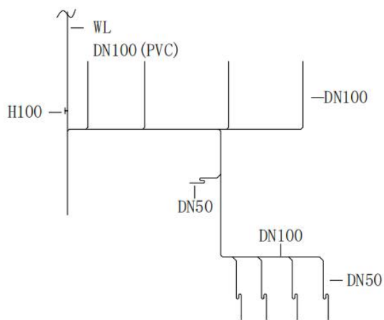
卫生间排水系统图
